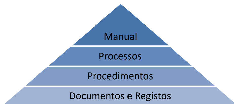
Figura 1 – Estrutura documental
